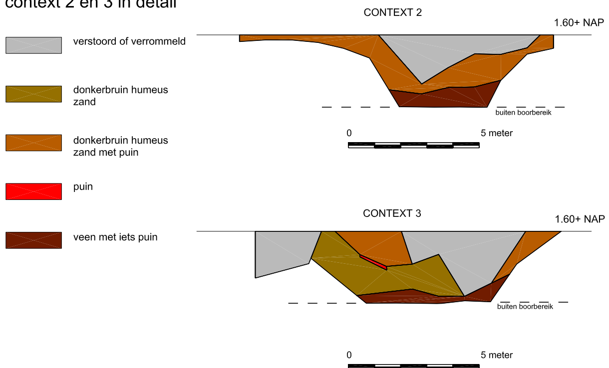
Afb. 12 Boorprofielen.
