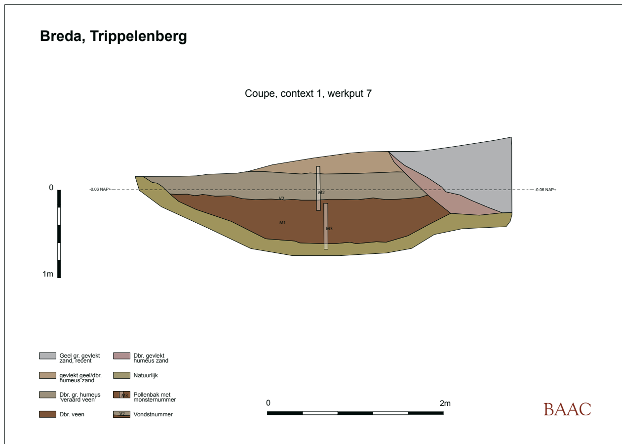
9.1 Tekening van de coupe door de gracht (context 1).
