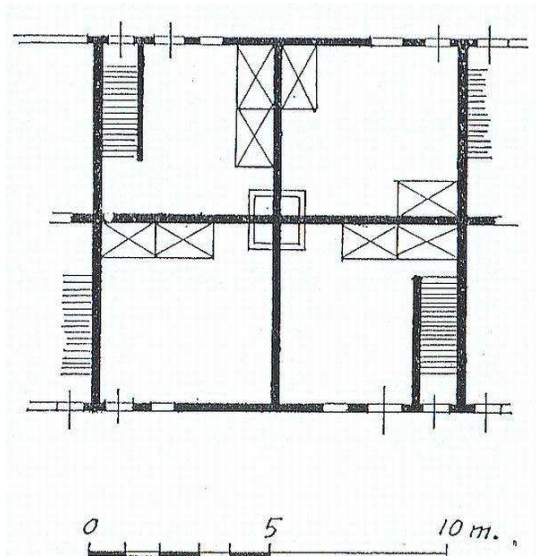
Afbeelding 10. Indeling barakken complex Akkerstraat
