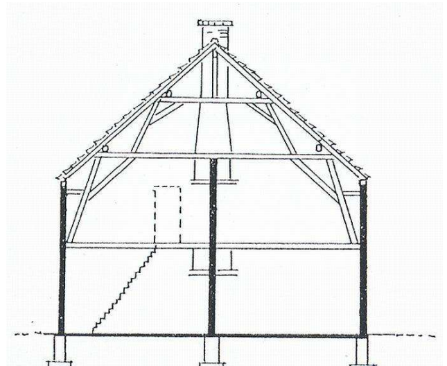
Afbeelding 11. Doorsnede barakken Akkerstraat
