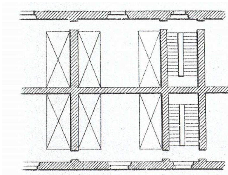
Afbeelding 6. Indeling barakkencomplex Givet
