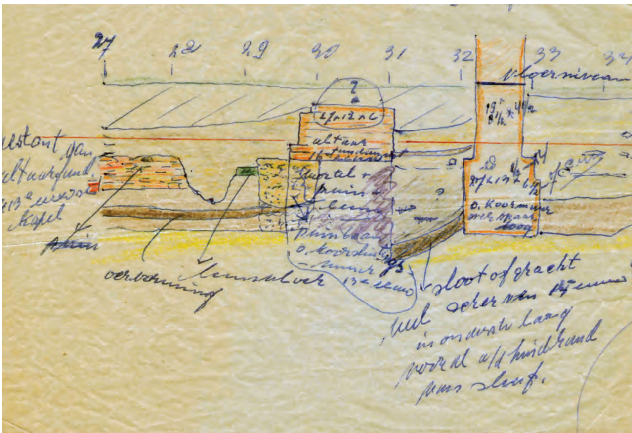
Afb.2.07: Deel van de profiel- tekening uit 1958.
