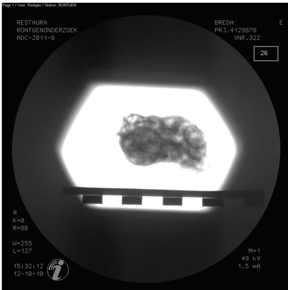
Afb. 8.15: Röntgenopname maliënkolder (Spoor 322, vnr. MT8062).
